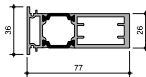
AW705 26mm Coupler
