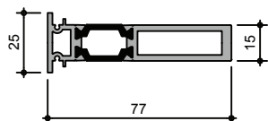
AW702 15mm Coupler
