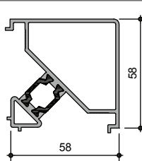
AW721 90° Bay Pole
